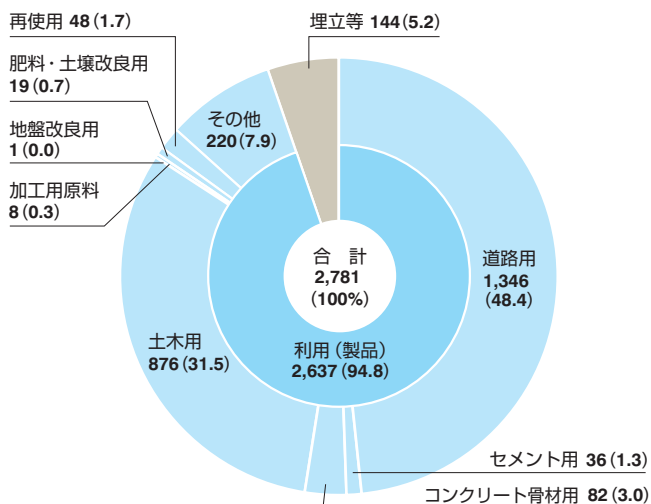
電気炉系スラグの用途別使用量
