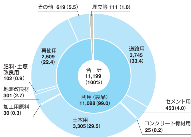
転炉系スラグの用途別使用量
