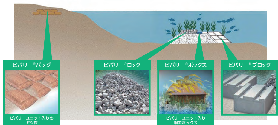
ビバリー®ユニット等の鉄鋼スラグ製品を利用した藻場造成のイメージ
