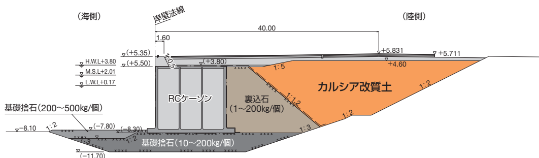
出断面図（東予港中央地区 耐震強化岸壁築造工事）
