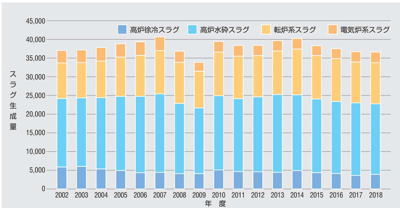
各種鉄鋼スラグの生産量推移
