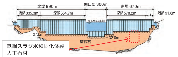
釜石湾口防波堤の側面図
