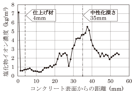
図 3. 塩化物イオン量と中性化深さ
