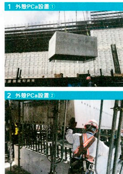
1 外殻PCa設置① 2 外殻PCa設置② 3 クリーンクリート打設 4 ガーダー架構完成
