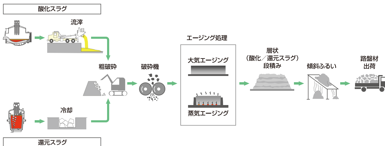
破碎・分級のフロー図（路盤材の製造工程例）
