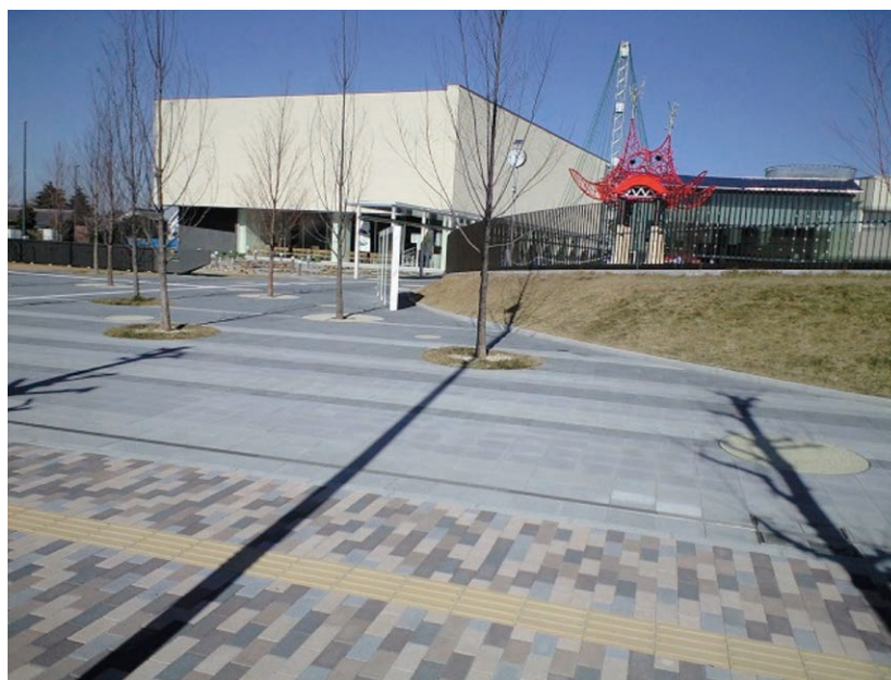
インターロッキングブロック使用例（豊橋市こども未来館） 〔粗骨材に EFG を 75% 混合〕
